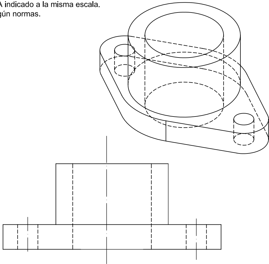
CORTE A-A
